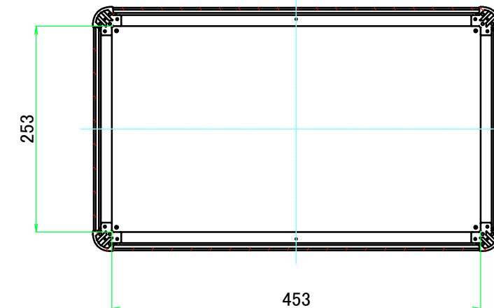
C-C ( 1 : 6.5 )
